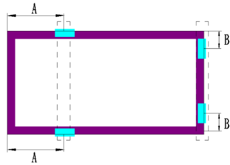
长短边四点混合安装
